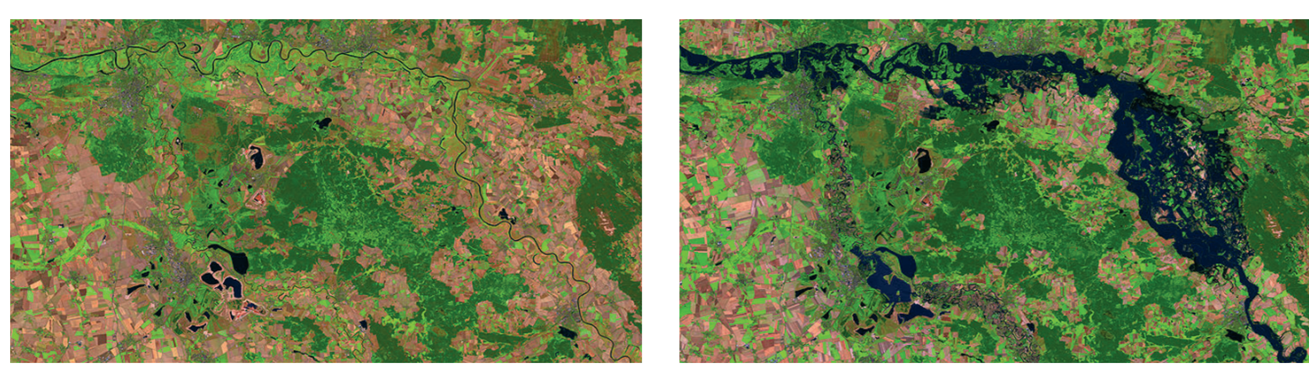
Abb. 2: Satellitenbilder der Elbe zwischen Torgau und Aken am 14. August 2002 und 20. August 2002 (während der Elbeflut). Quelle: NASA. https://upload.wikimedia.org/wikipedia/commons/a/a8/NASA_Elbe_flood_2002_before_after.jpg
