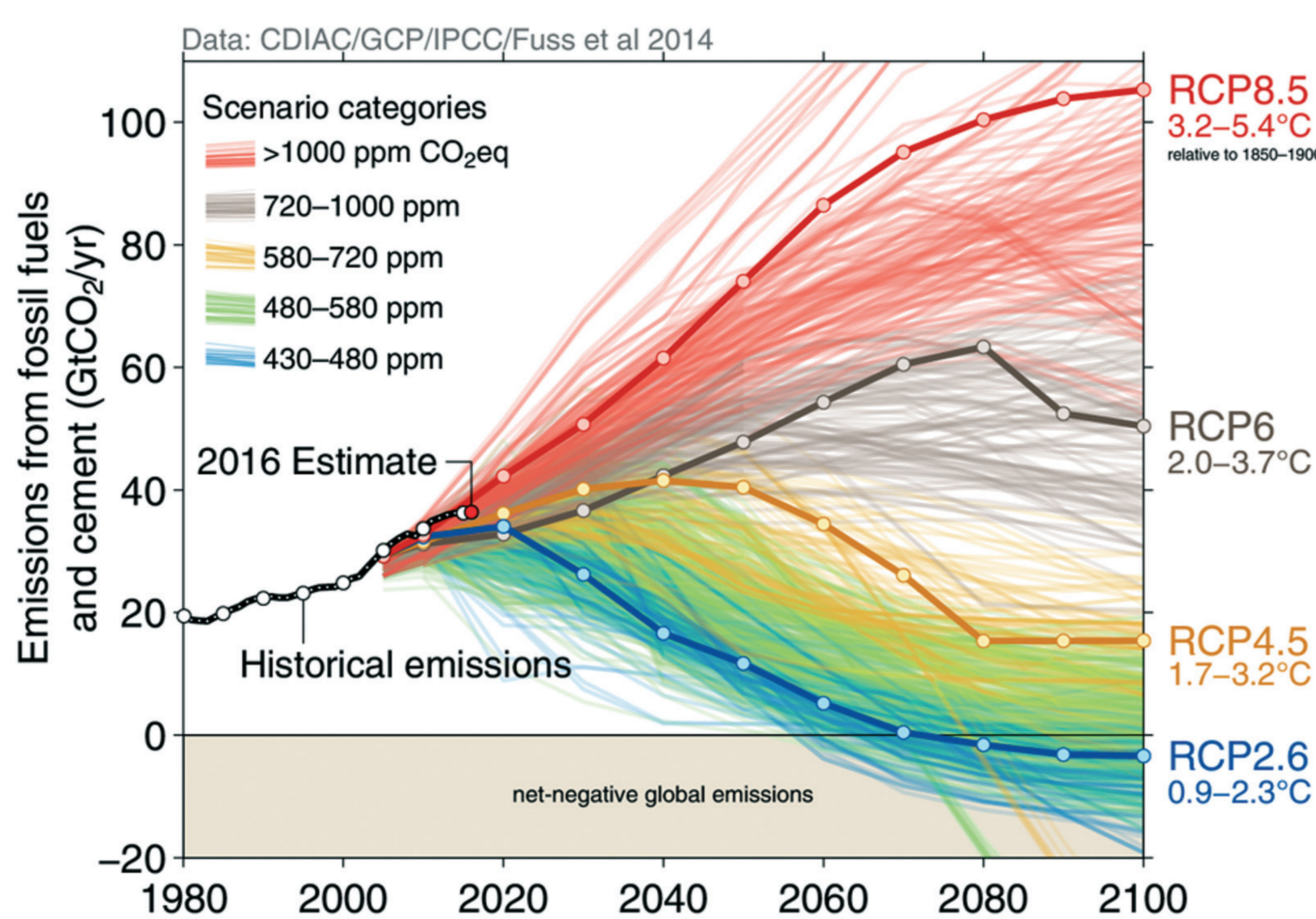
Abb. 1: Emissionsszenarien des Weltklimarats IPCC. (vgl. grauer Kasten rechts). Auf der y-Achse sind die jährlichen CO 2 -Emissionen in Mrd. t (ohne Landnutzungsänderungen) angegeben.
