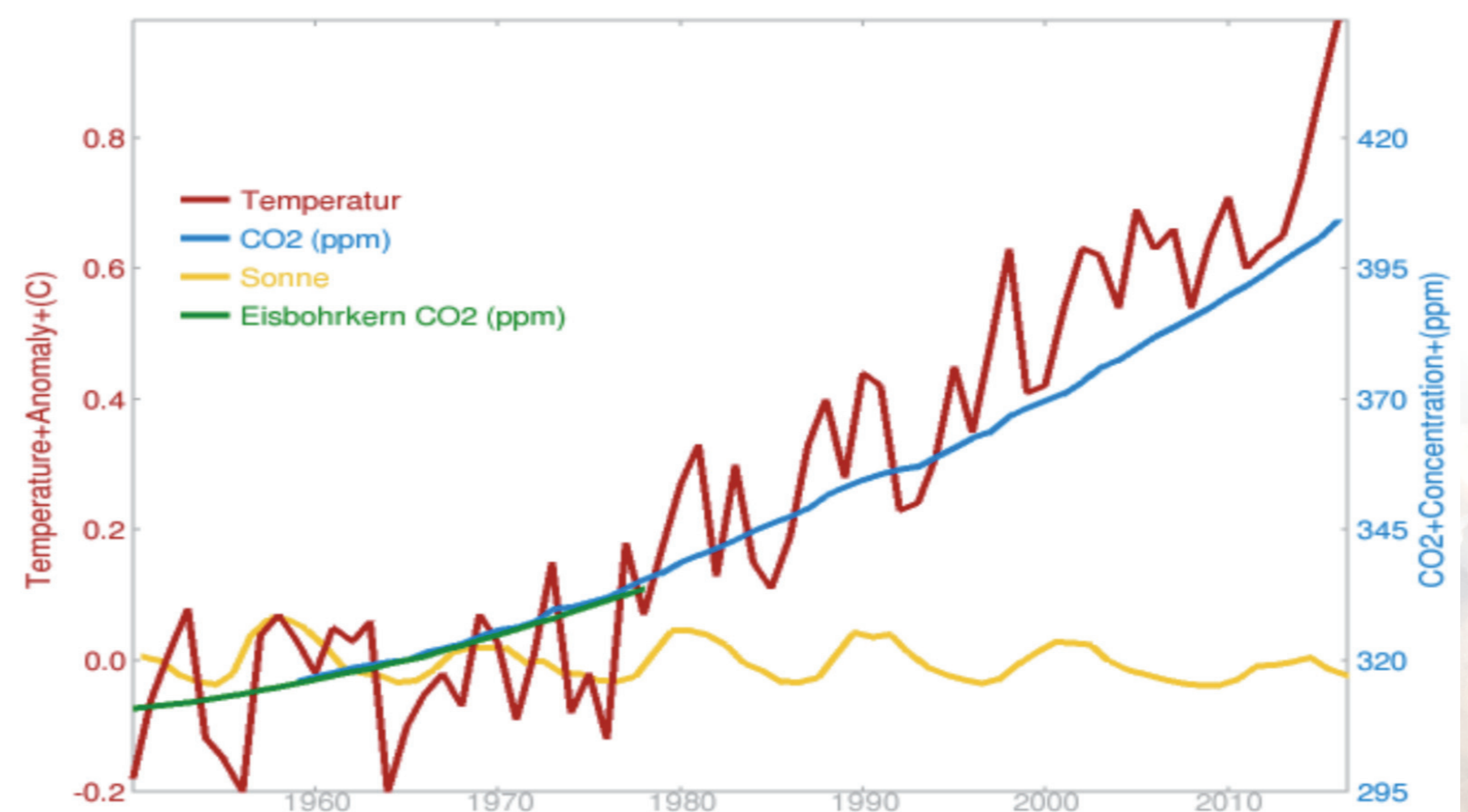
Abb. 2: Verlauf von globaler Temperatur, CO 2 -Konzentration und Sonnenaktivität ab 1950 bis 2015. http://scllogs.spektrum.de/klimalounge/files/need_widget-1.png
