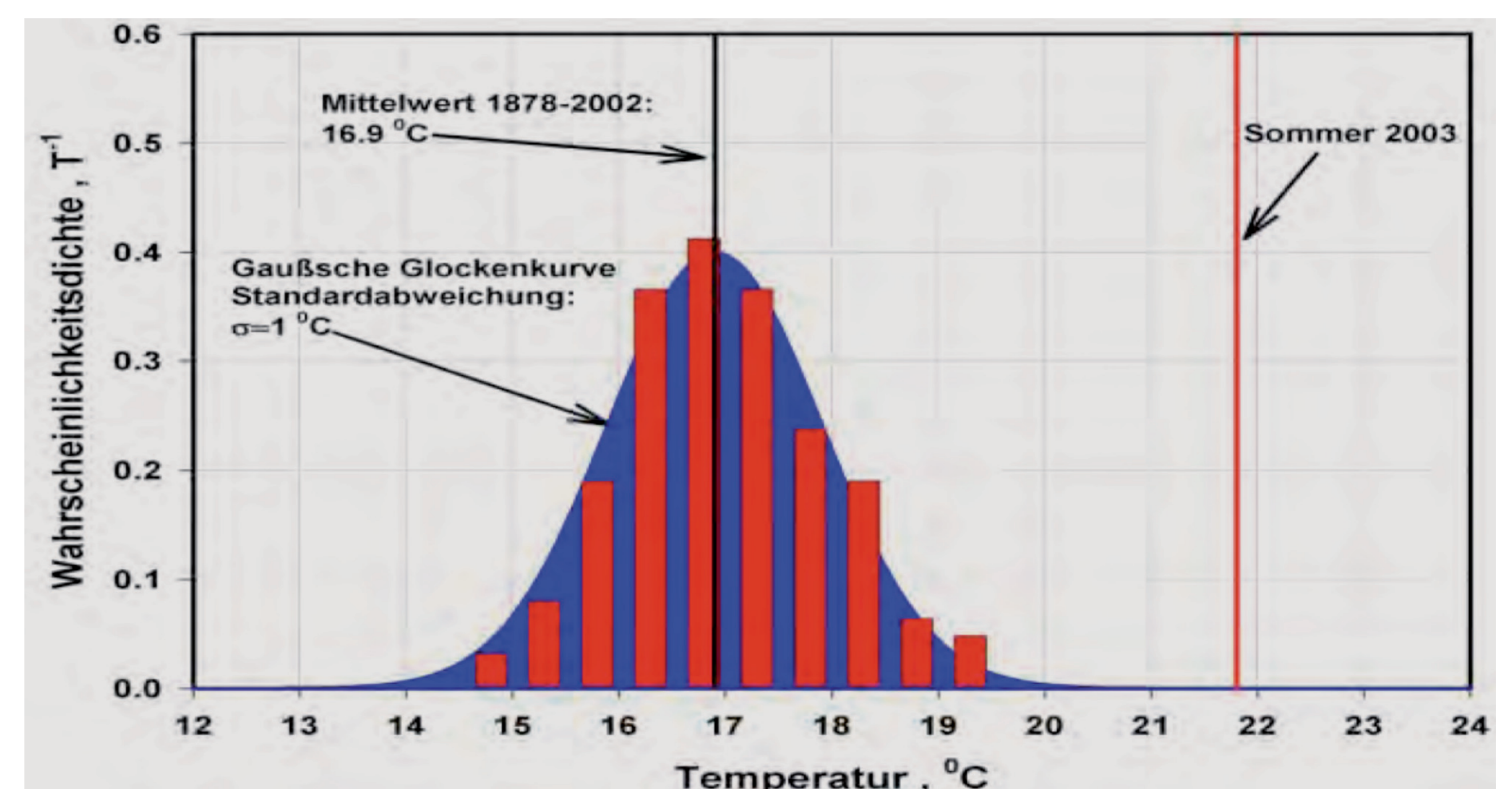
Abb. 2 Verteilung der Sommertemperaturen in Stuttgart-Hohenheim 1878 – 2003.
